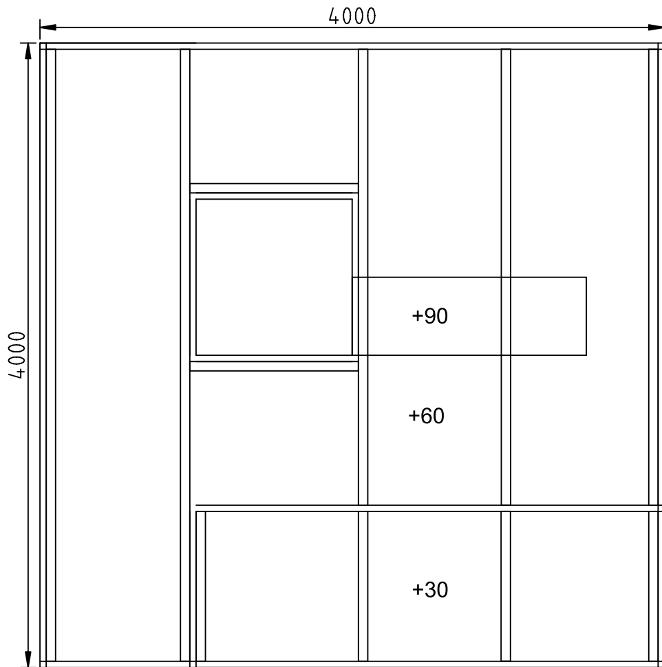
Unterzüge , Pfosten Lärche 60/120
