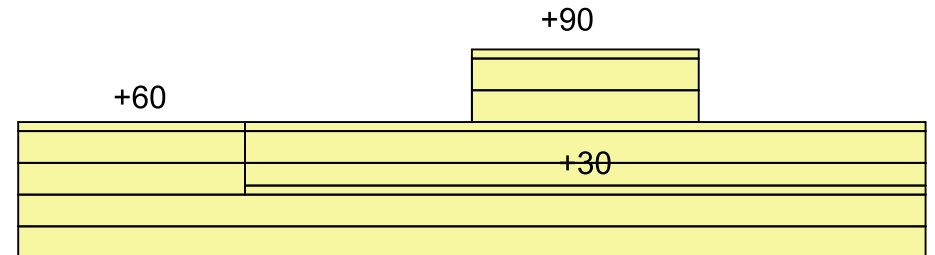
Belag und Seitenverkleidung Lärche 40/140
